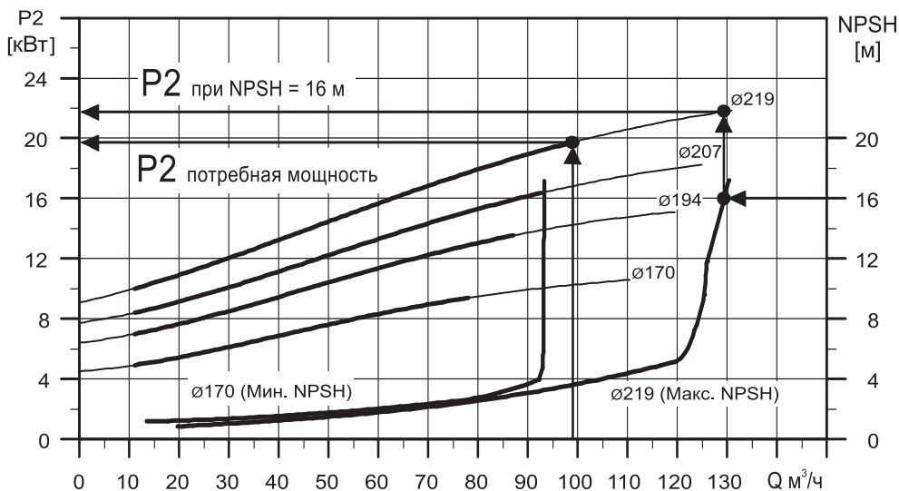
Рис. 6 Расчет мощности двигателя. Потребная мощность P2: 22 кВт, минимальная необходимая мощность двигателя с учетом запаса 10%: 22 кВт + 10 % = 24,2 кВт.
