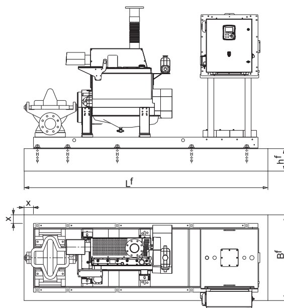
Рис. 5 Размеры основания
