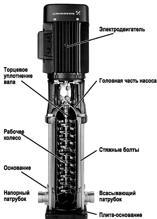
Рис. 6 Жокей-насос
