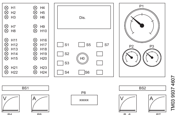
Рис. 16 Панель управления
